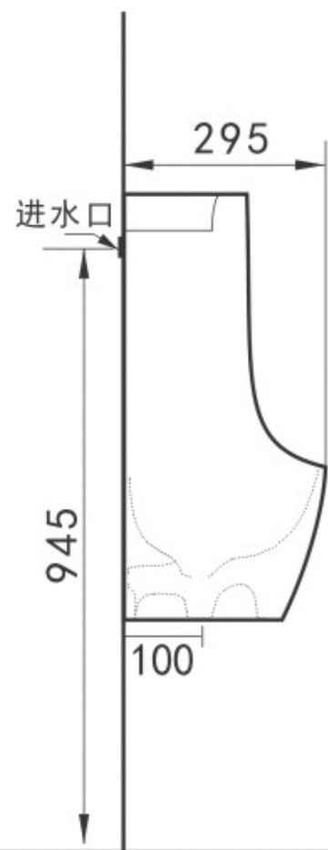
直排水
