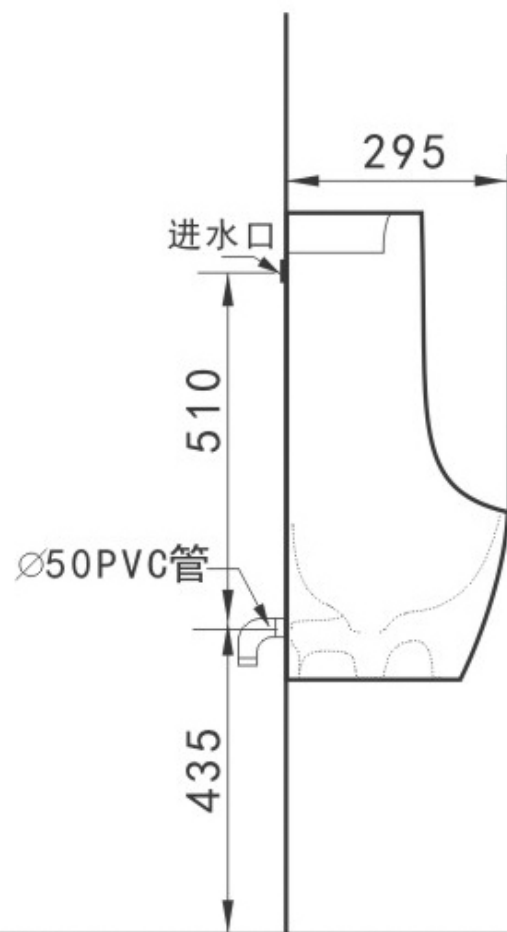
墙排水
